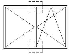
A = Fori di fissaggio P.1202 con P.1233 A = Anchoring holes P.1202 with P.1233
