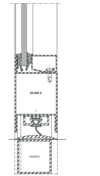
Barrier-free door
