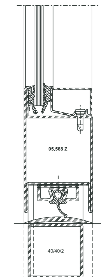
Barrier-free door
