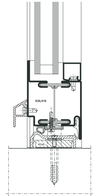
Barrier-free door
